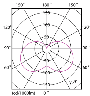
LEDbulb 60W E14 827 FR B38
