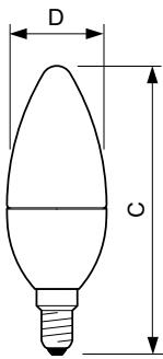
Candle 230V 8-60W 806lm 2700K E14 ND FR
