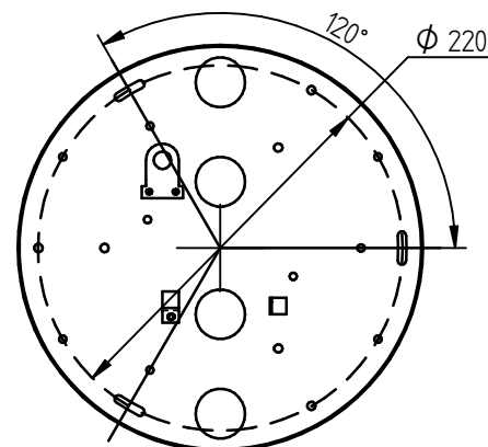
Bohrschablone
