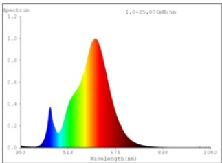
VALGL9575 7,5W 827
