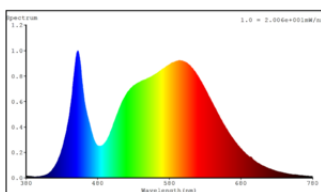
VALCLB75 7,5W 840 GLFR E27
