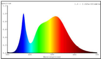
VALCLP75 7,5W 840
