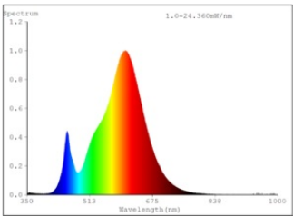
VALCLB75 7,5W 827 GLFR
