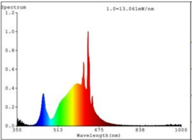
VALUE CLB25 2,8W 830
