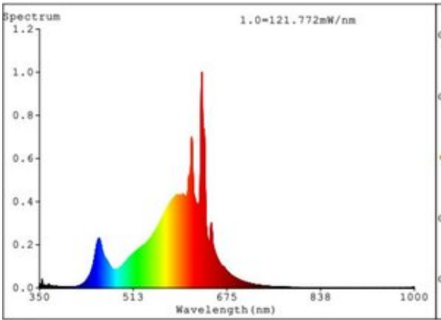
VALUE CLA150 19W 827
