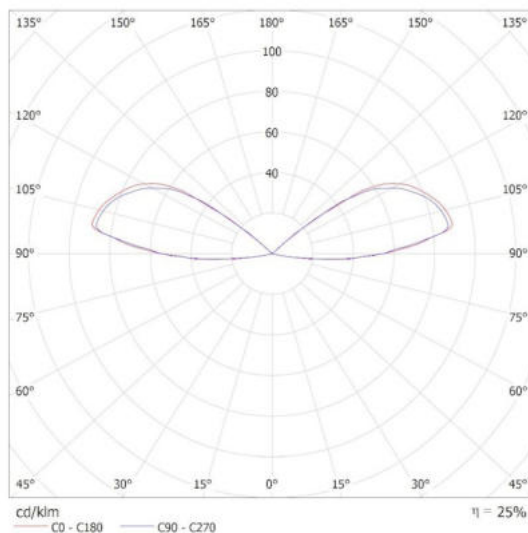
KANLUX S.A. (kat 39181) REFAZI EL 6W-F-GR / Krzywa rozsyłu światła (biegunowo)
