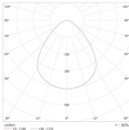
KANLUX S.A. (kat 39171) BLINGO UHRA 95 120NW / Krzywa rozsyłu światła (biegunowo)
