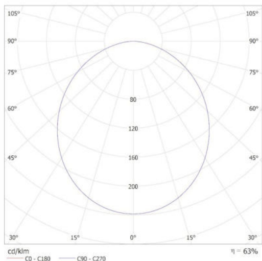
KANLUX S.A. (kat 39026) DABER 12-20W CCT B 12W / Krzywa rozsyłu światła (biegunowo)
