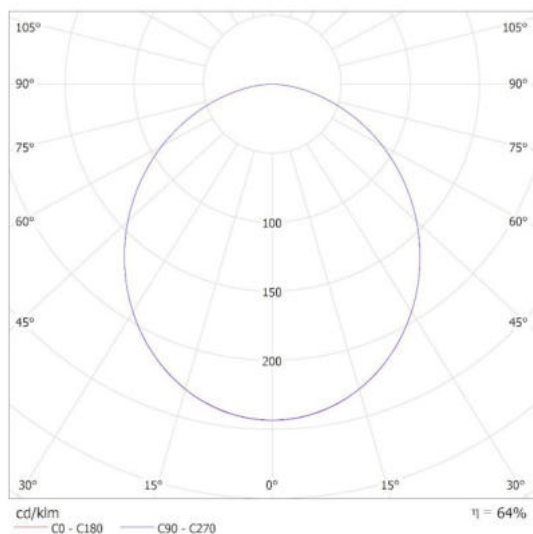
KANLUX S.A. (kat 39024) DABER 12-20W CCT W 12W / Krzywa rozsyłu światła (biegunowo)
