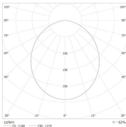
KANLUX S.A. (kat 39021) DABER 8-13W CCT SE W 8W / Krzywa rozsyłu światła (biegunowo)
