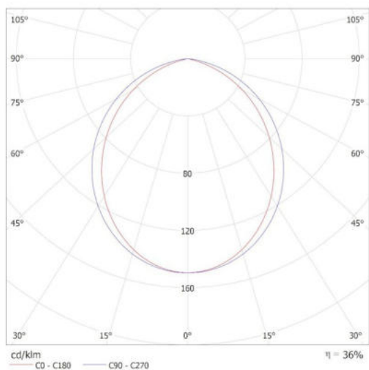
KANLUX S.A. (kat 38895) YALTE D 09 8W WW-B / Krzywa rozsyłu światła (biegunowo)
