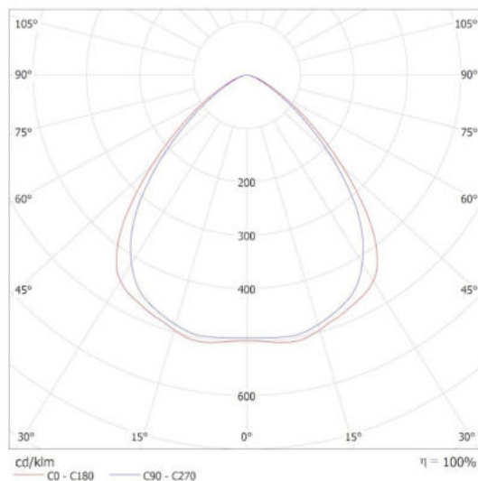
KANLUX S.A. (kat 36602) IQ-LEDEX GU10 4,7W-NW / Krzywa rozsyłu światła (biegunowo)
