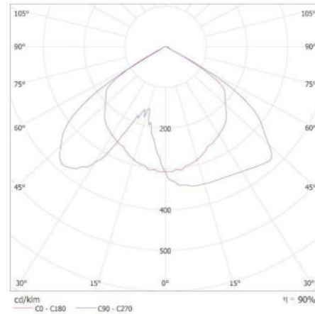
KANLUX S.A. (kat 36435) PARCOLI 30-50W CCT G_30st / Krzywa rozsyłu światła (biegunowo)
