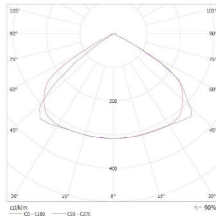
KANLUX S.A. (kat 36435) PARCOLI 30-50W CCT G_60st / Krzywa rozsyłu światła (biegunowo)
