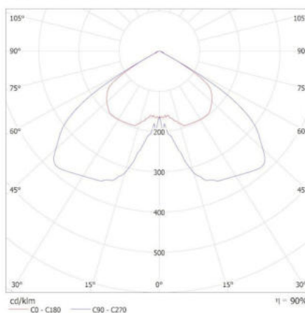
KANLUX S.A. (kat 36435) PARCOLI 30-50W CCT G_0st / Krzywa rozsyłu światła (biegunowo)
