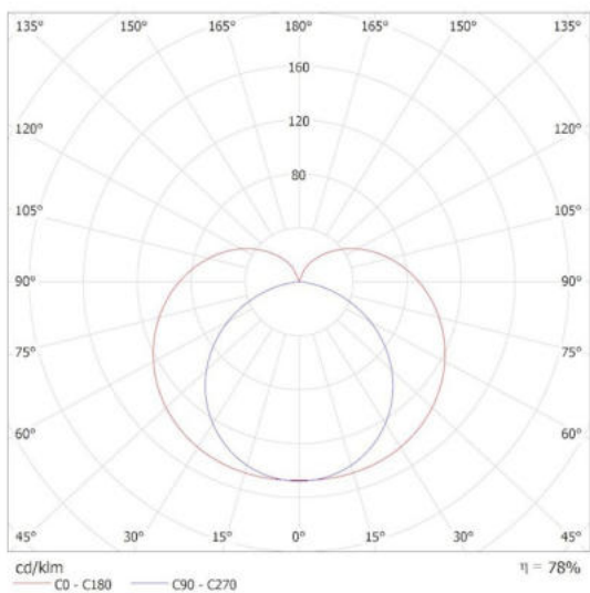
KANLUX S.A. (kat 29217) MERA LED 11W CCT / Krzywa rozsyłu światła (biegunowo)
