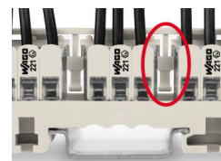
Einbauweise 440 V Positionierung der Klemmen im Adapter mit Distanzelement zwischen den Klemmen
