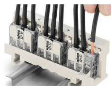
Lösen der Leiter im Befestigungsadapter
