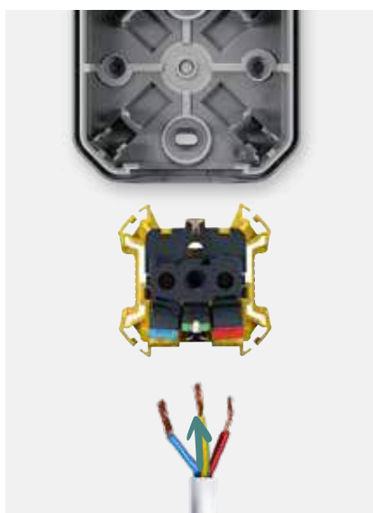
Mechanismus ist nicht eingerastet am Grundkörper
